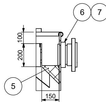
SEZIONE F-F SCALA 1 : 20
