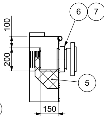
SEZIONE F-F SCALA 1 : 20
